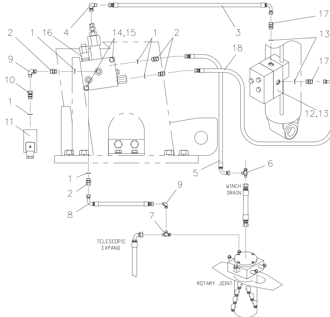
로드 리미트 배관 Fig. 5-7 SCS323 LOAD LIMMIT PIPING
