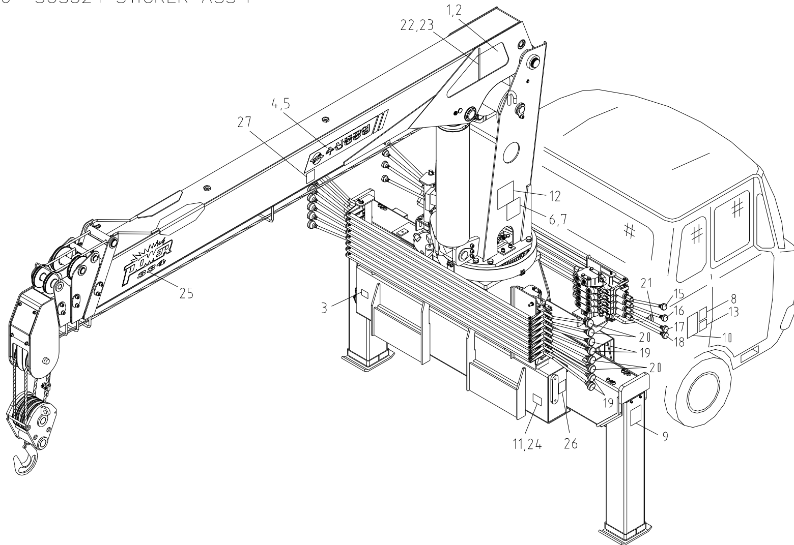
스티커 조립체 Fig. 6 SCS324 STICKER ASS'Y
