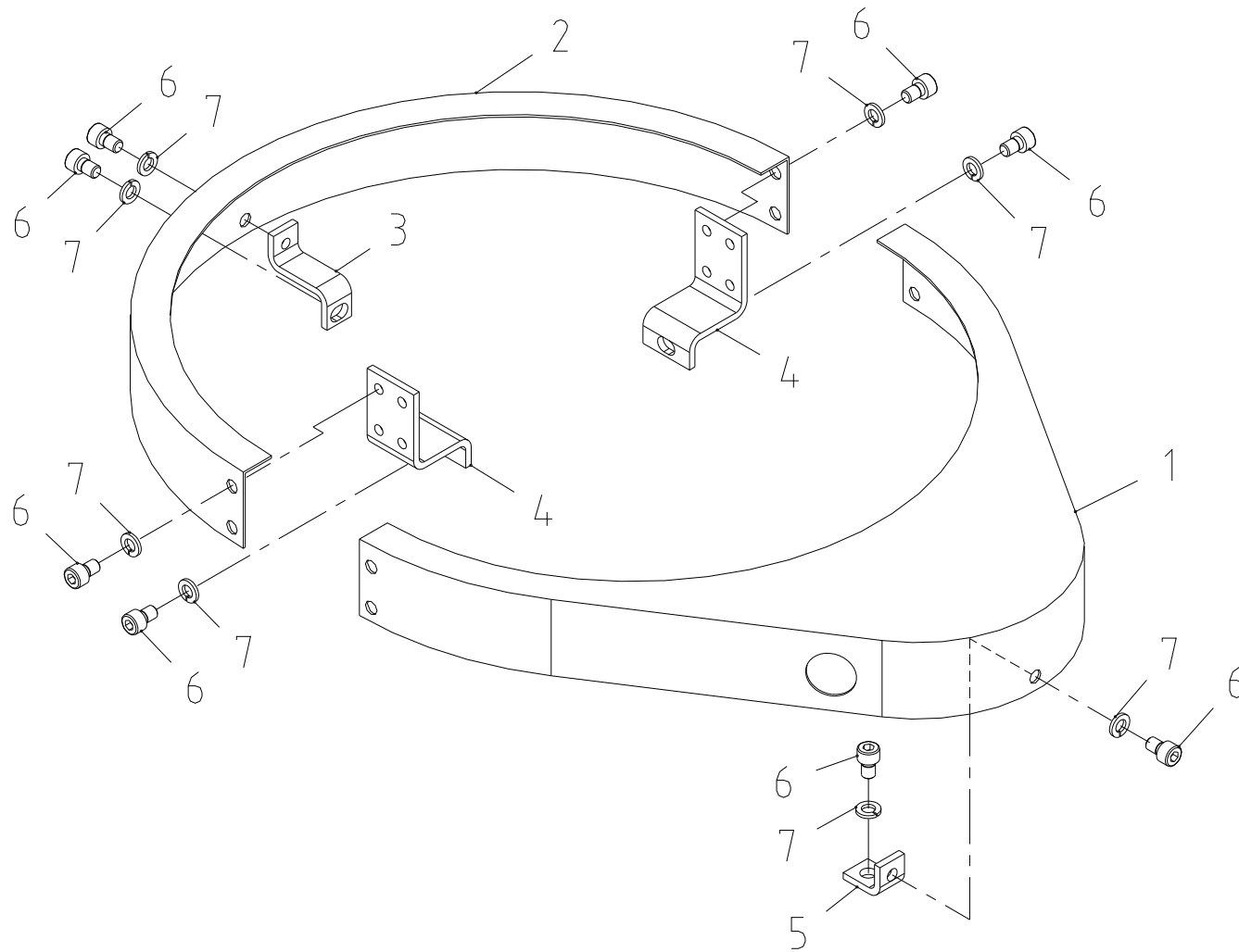
기어 커버 조립체 Fig. 3-3 SCS323 GEAR COVER ASS'Y
