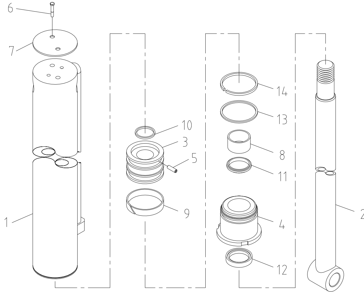
잭 실린더 조립체 Fig. 4-1 SCS323 JACK CYL' ASS'Y
