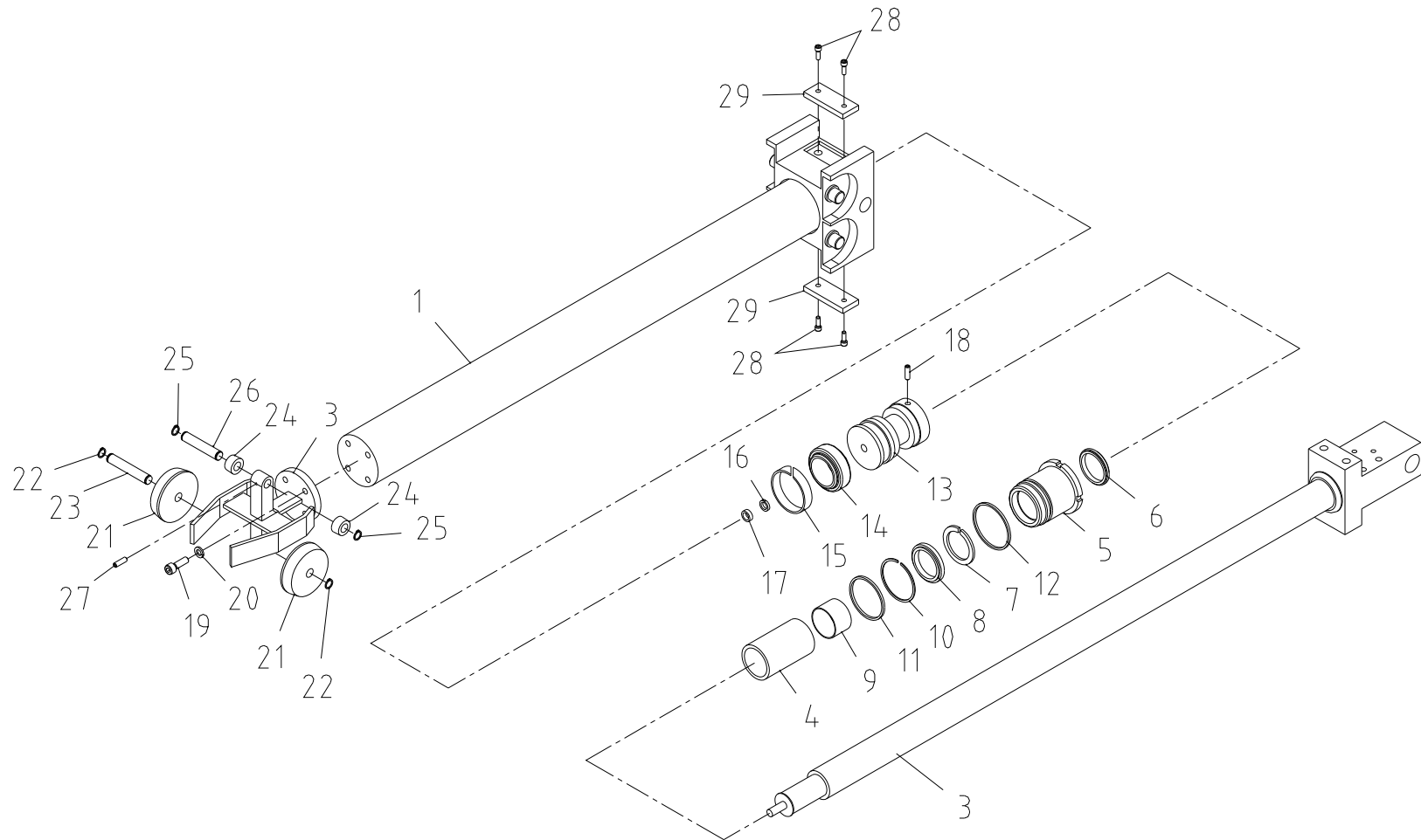
텔레실린더 조립체 Fig. 1-1 SCS323 TELE' CYL' ASS'Y
