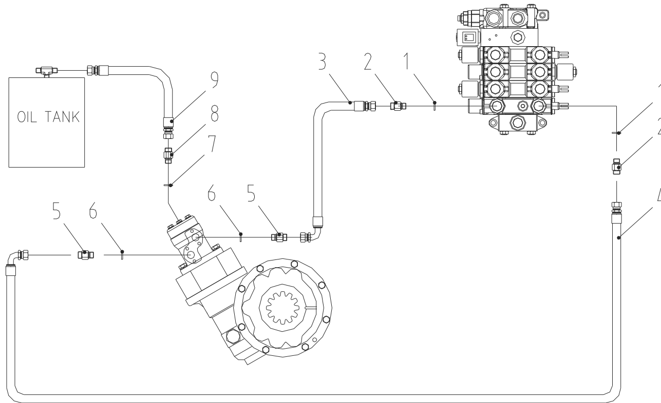
스윙 배관 Fig. 5-5 SCS323 SWING PIPING
