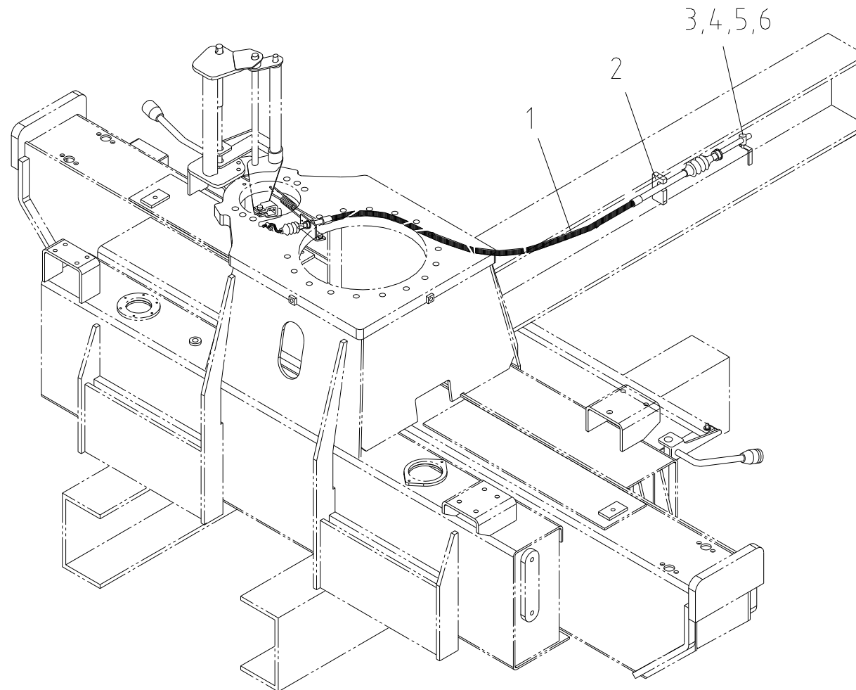
악셀 시스템 파트 Fig. 8-3 SCS323 ACC' SYSTEM PART
