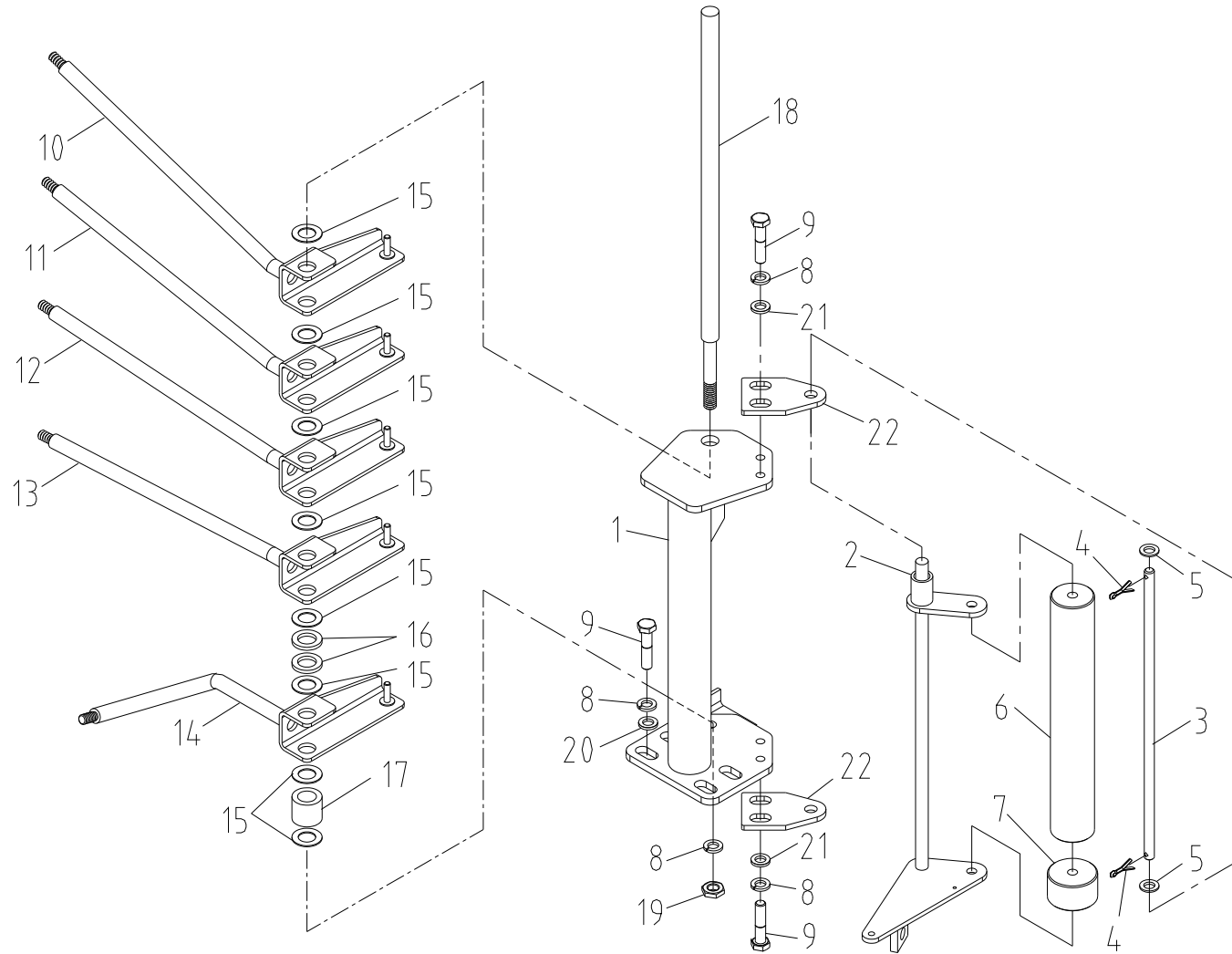
레버 스텐드 셋 Fig. 3-5-2 SCS323 LEVER STAND SET
