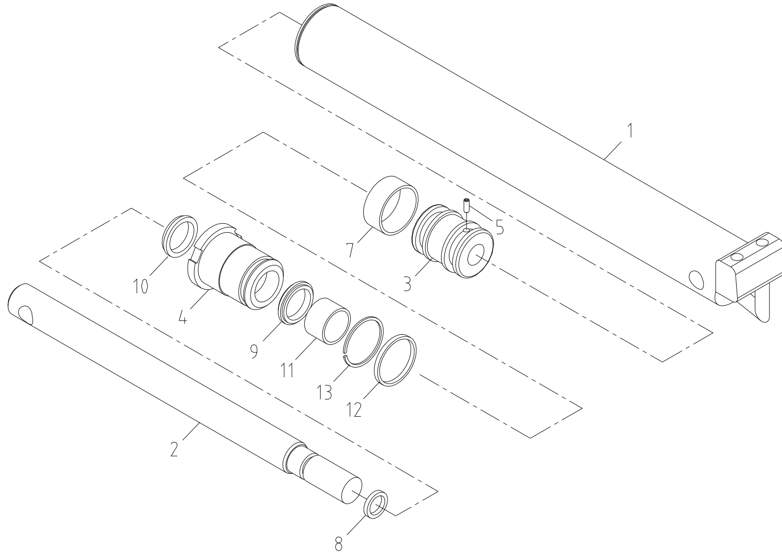
익스펜드 실린더 조립체 Fig. 4-2 SCS323 EXPAND CYL' ASS'Y
