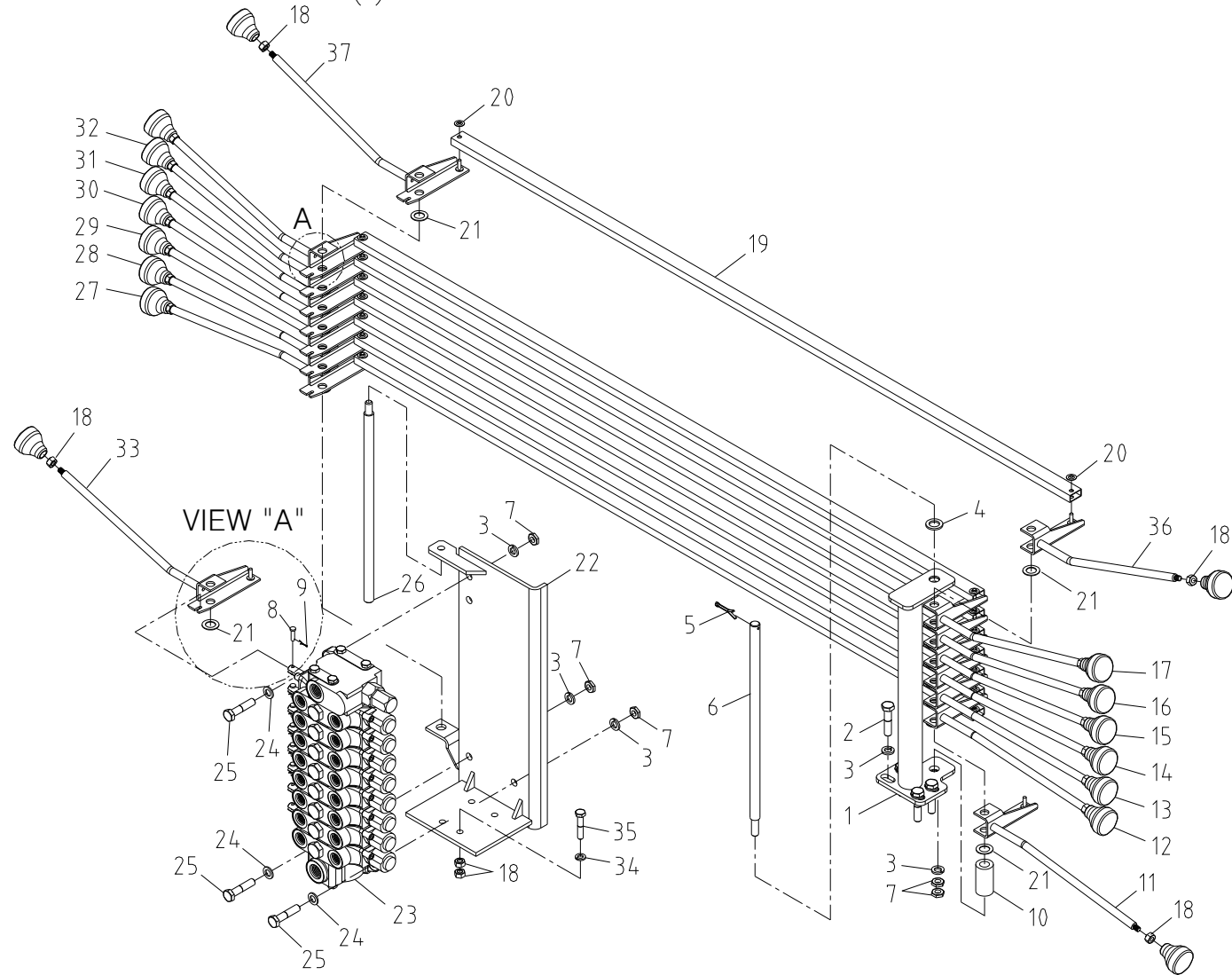
오퍼레이션 조립체 (I) Fig. 3-4 SCS323 OPERATION ASS'Y(I)
