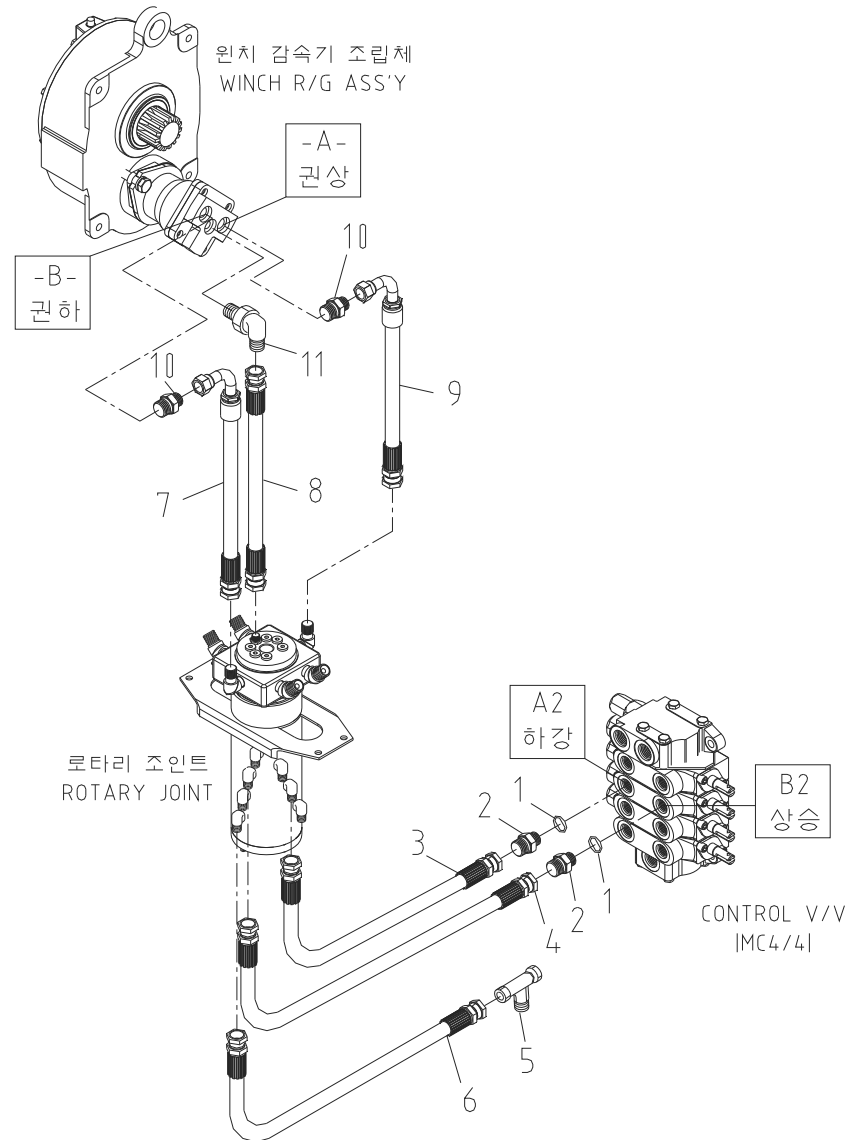
원치 배관 Fig. 5-3 SCS323 WINCH PIPING
